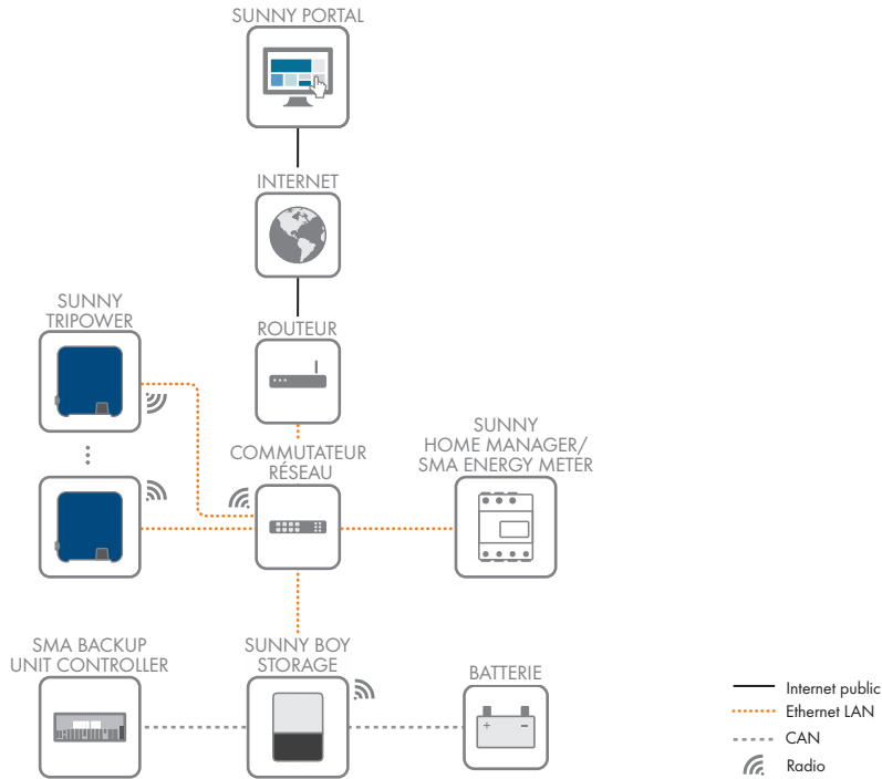
Figure 5 : Établissement communication
