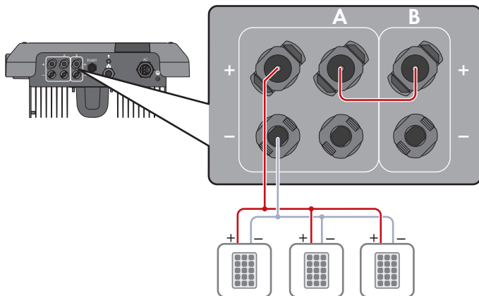
Figure 11 : Vue d'ensemble du raccordement en montage en parallèle des entrées DC A et B
