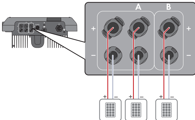
Figure 10 : Vue d'ensemble du raccordement en fonctionnement normal
